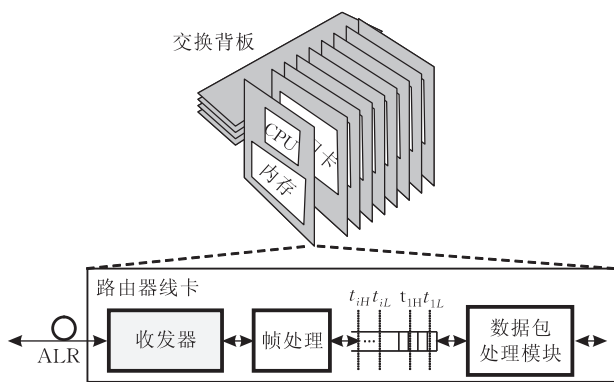
图 1 路由器线卡中各个模块之间通存队列相连
