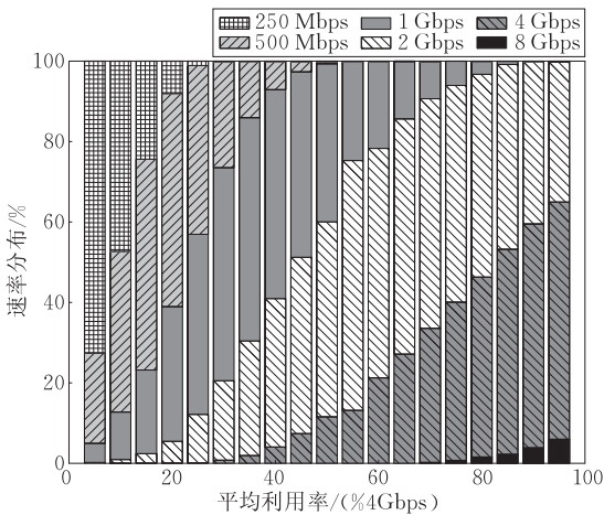
图 10 B 组指数阈值配置在不同负载下的平均速率分布
