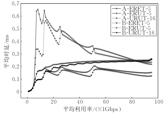
图 4 不同分布、阈值在不同负载下的平均时延
