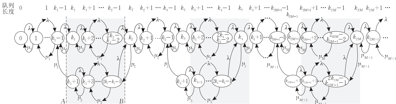
图 3 多双阈值的马尔科夫链
