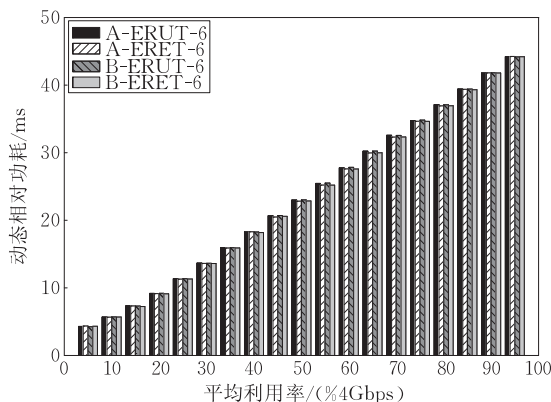
图 9 应用 FASS 的模块在不同负载下的动态相对功耗
