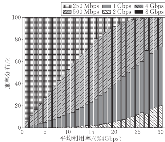
图 11 B 组指数阈值配置在 1%~30% 负载下的平均速率分布
