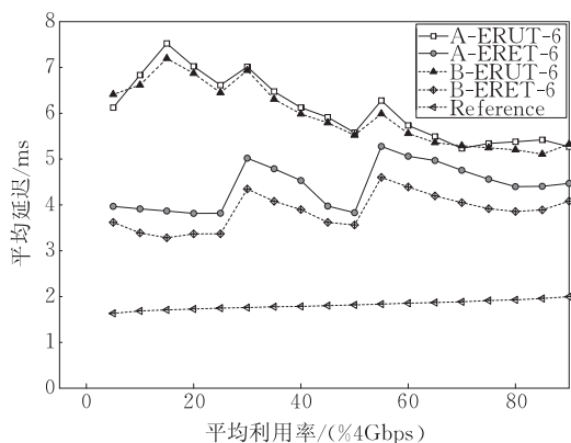
图 8 参考路由器和 FASS 路由器在不同配置、不同负载下的时延
