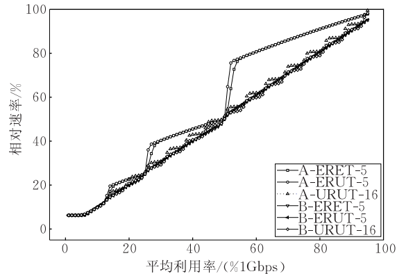
图 5 不同分布、阈值在不同负载下的相对速率
