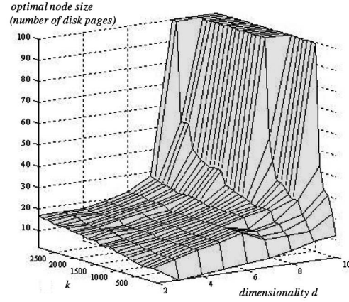
Fig. 9. Optimal node sizes (disk page = 1k bytes).
