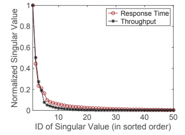
Fig. 9. Sorted Singular Values
