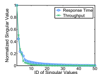
Fig. 9. Sorted Singular Values
